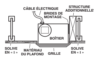
BOÎTIER MONTÉ SUR UNE SOLIVE EN « I » Nécessite une structure additionnelle pour les brides de montage. Évacuation parallèle aux solives.
