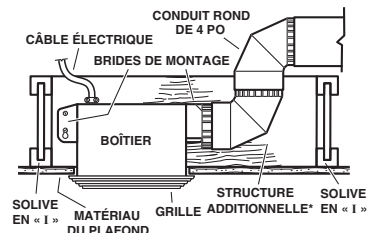
BOÎTIER MONTÉ SUR UNE SOLIVE EN « I » Nécessite une structure additionnelle pour les brides de montage. Évacuation à 90° des solives.
